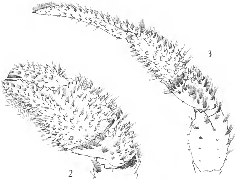
FIG. 2, 3. — Dardanus brachyops sp. nov., ♂ holotype. 2, région distale du chélicède gauche ( \times 1 ). 3, troisième patte thoracique gauche ( \times 0,75 ).
